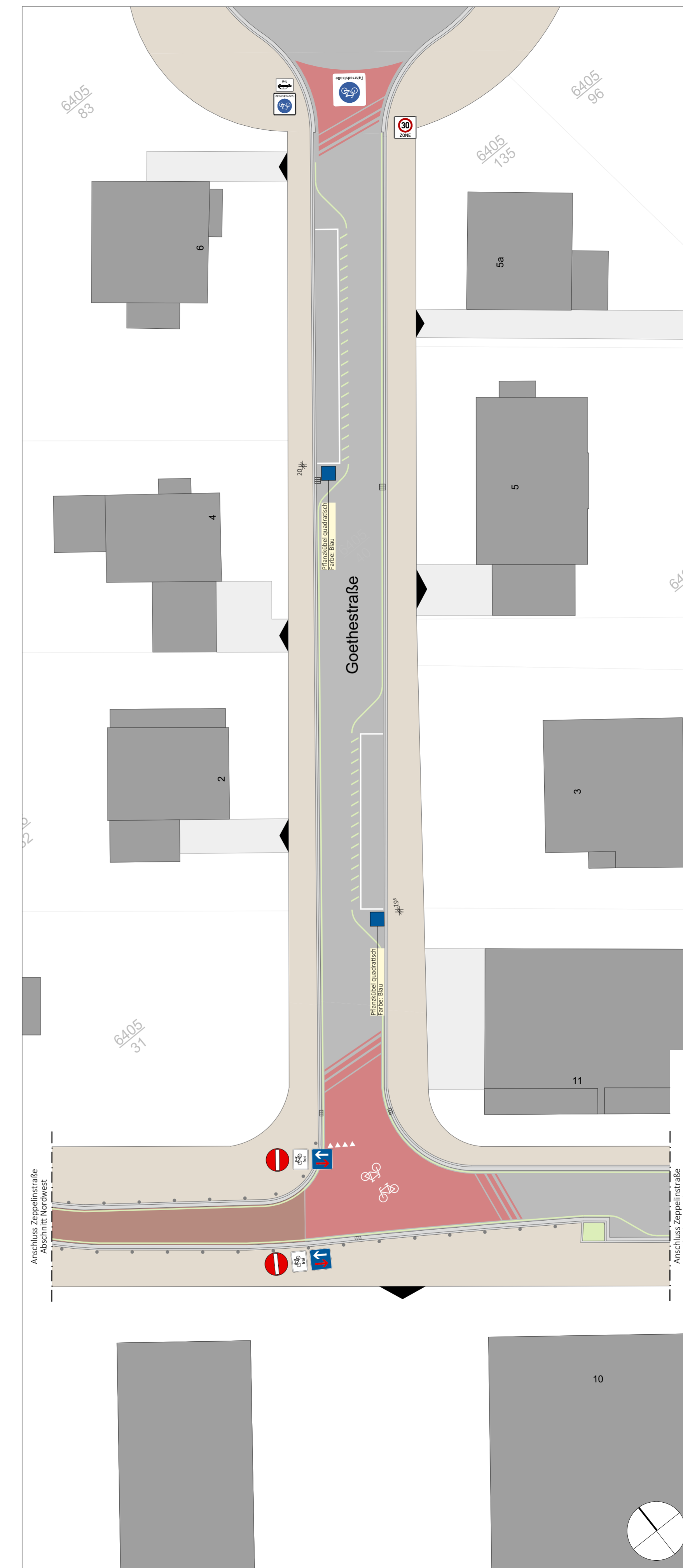
Goethestraße / Zeppelinstraße Abschnitt Mitte M 1:250
