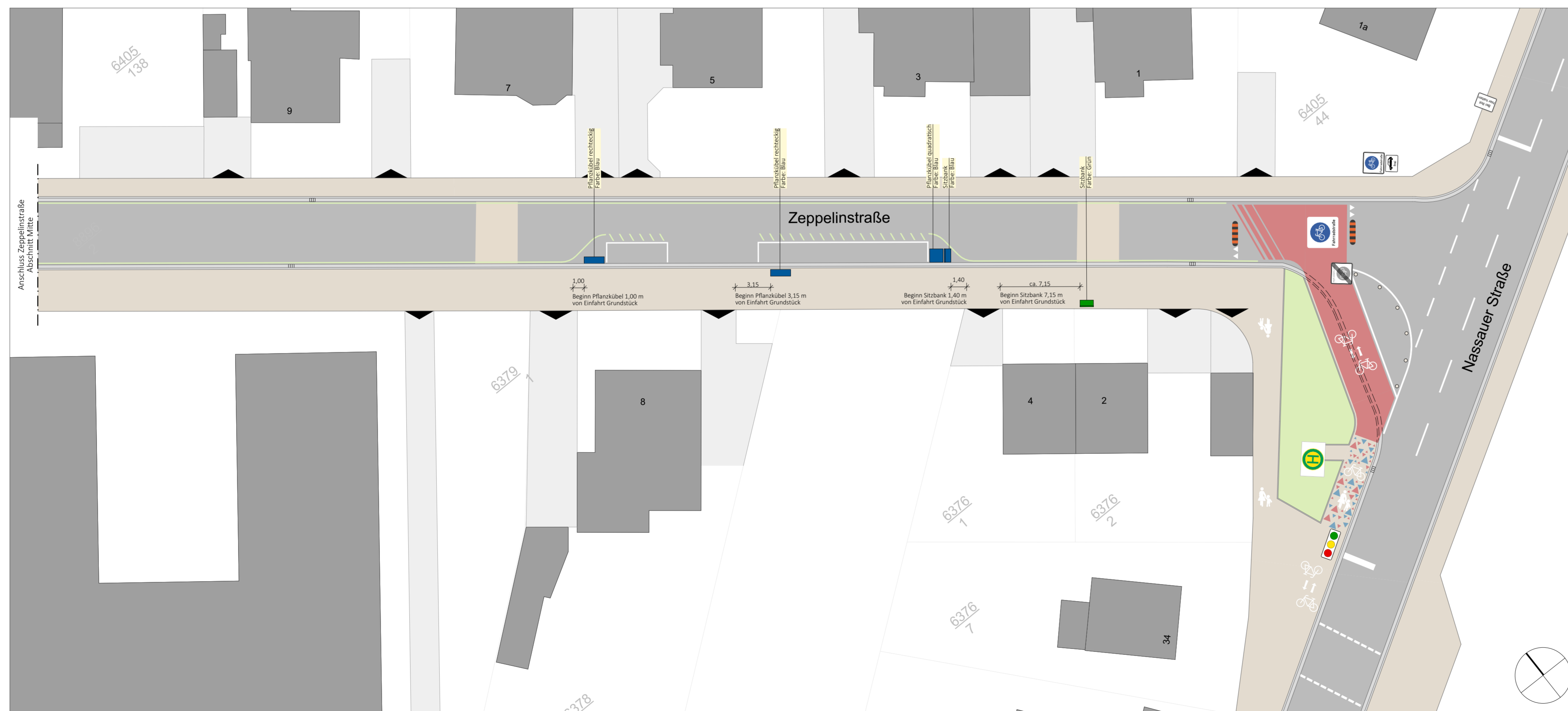
Zeppelinstraße Abschnitt Südost M 1:250
